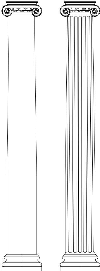
COLONNA/PARASTA IONICA
