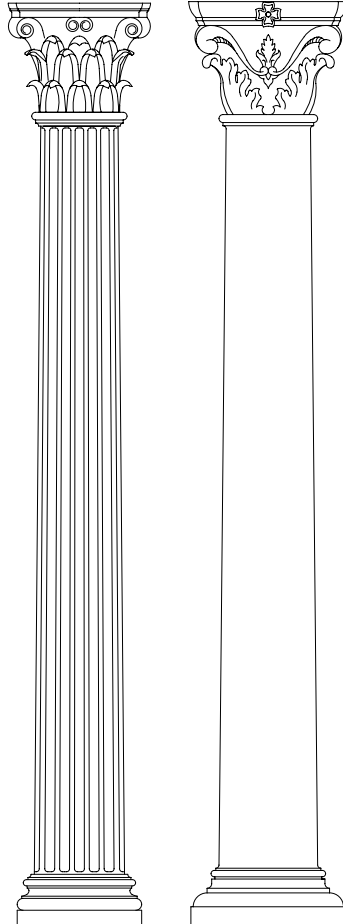
COLONNA/PARASTA CORINZIA
